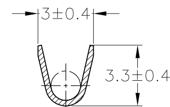
断面 A-A SECT A-A
