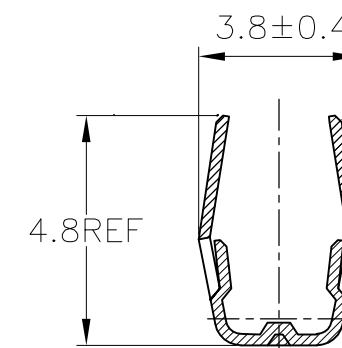
断面 B-B SECT B-B (175030のみ適用) (ONLY 175030)
