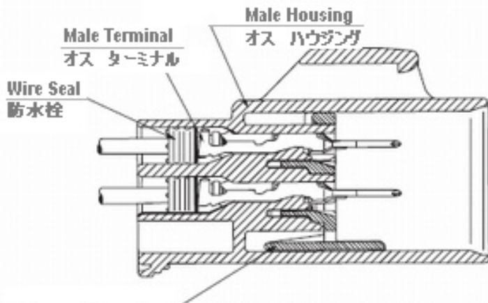
Male Pre-set Secondary Terminal Lock(TPA) オス側 事前組付け二重係止板
