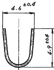
断面 B-B
