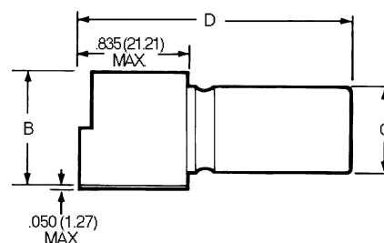
Receptacle
