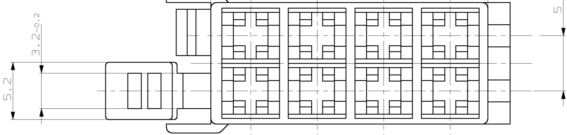
Schnitt A-B um 90° gedreht
