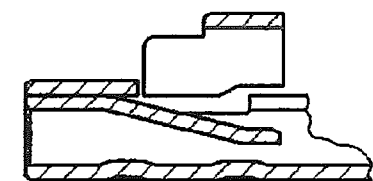
断面 "A" - "A" (SECT) (175152-1, -2, -3)
